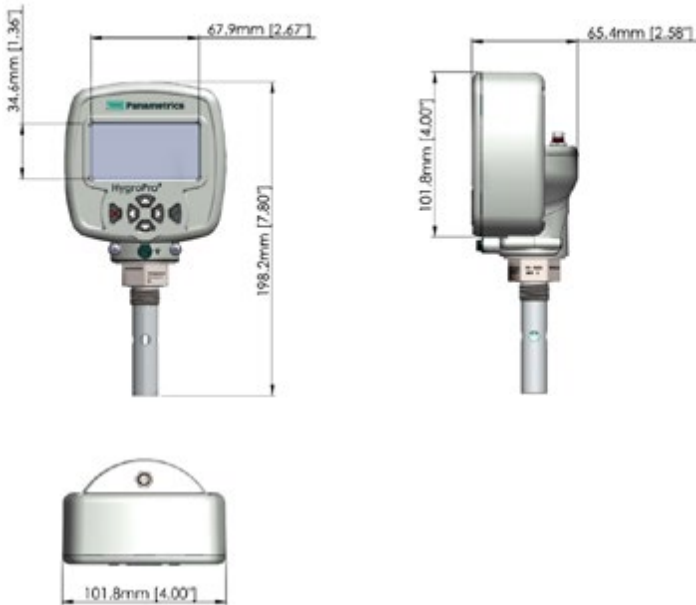
HygroPro ® dimensions
